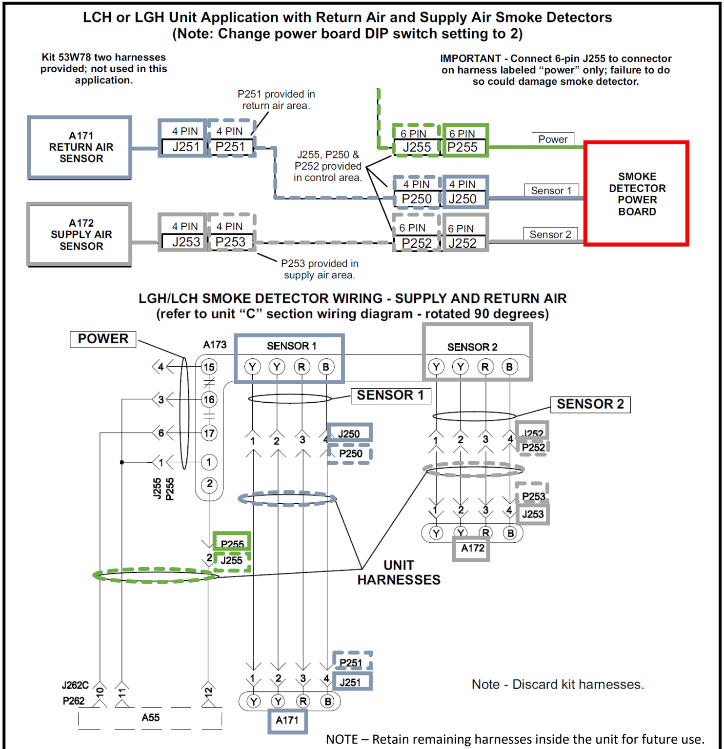
Figure 2. Schémas de raccordement provenant du manuel 506218
