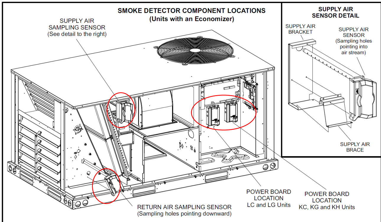
Figure 1. Emplacement des composantes de détection de fumée
